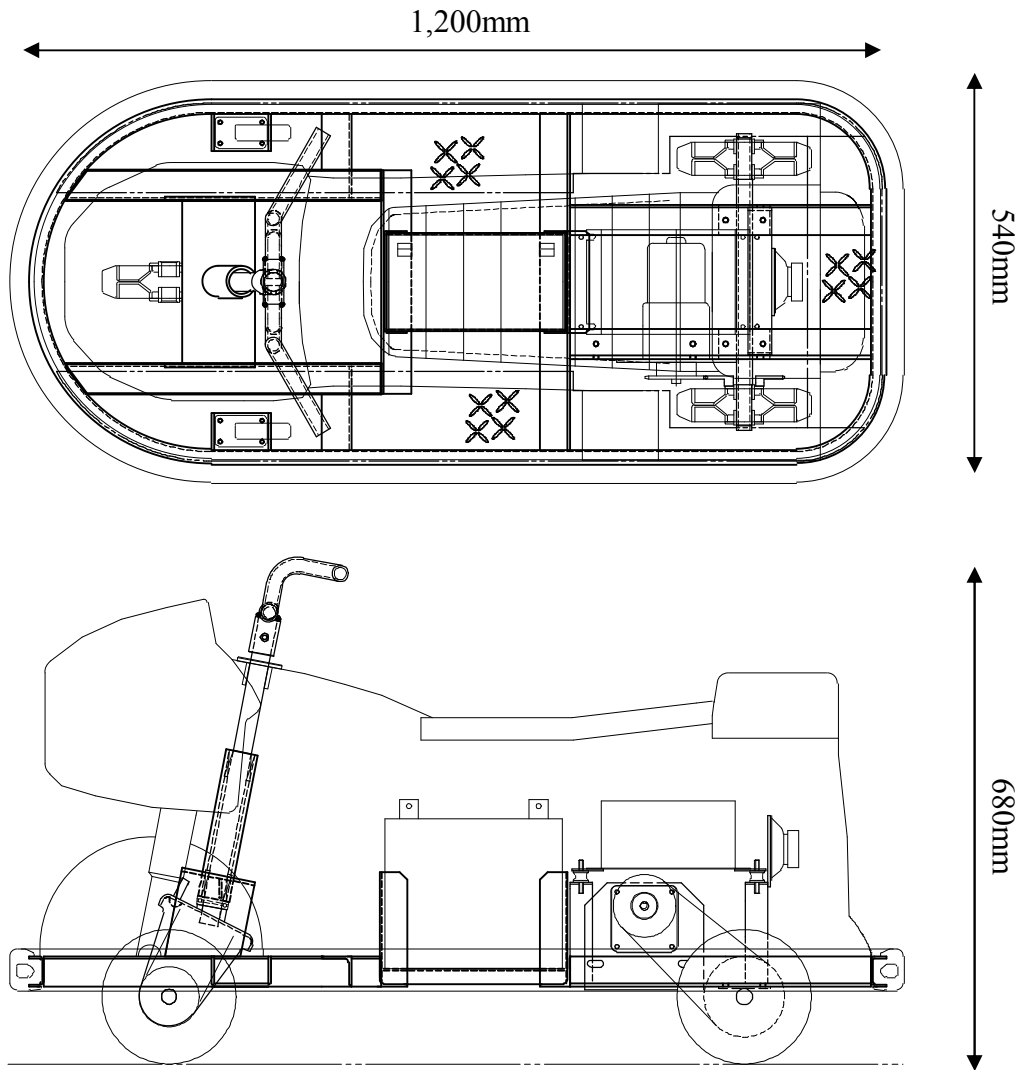
外形寸法図
